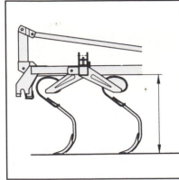
VF 2000/4200/4300/4000 Frigångshöjd m. VF-pinne: 75 cm Frigångshöjd m. VFM-pinne: 85 cm
